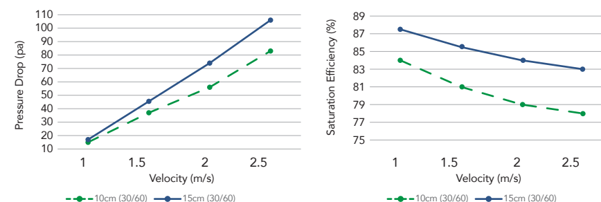
نمودار راندمان و افت فشار سری ۵۰۹۰ (۳۰/۶۰)
