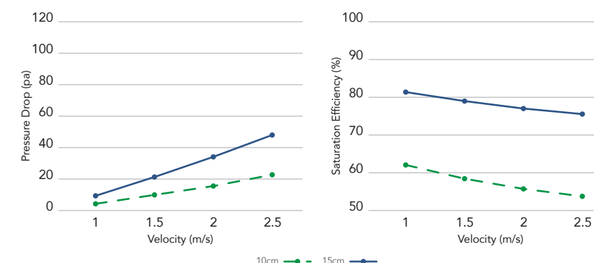
نمودار راندمان و افت فشار سری ۷۰۶۰
