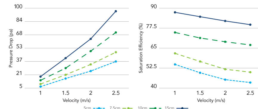
نمودار راندمان و افت فشار سری ۷۰۹۰ (۴۵/۴۵)
