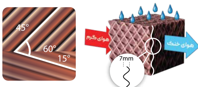
شکل ۵: مشخصات پد ۷۰۶۰
