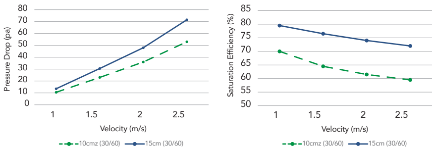
نمودار راندمان و افت فشار سری (۳۰/۶۰) ۷۰۹۰
