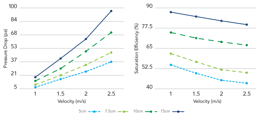
نمودار راندمان و افت فشار سری (۴۵/۴۵) ۷۰۹۰
