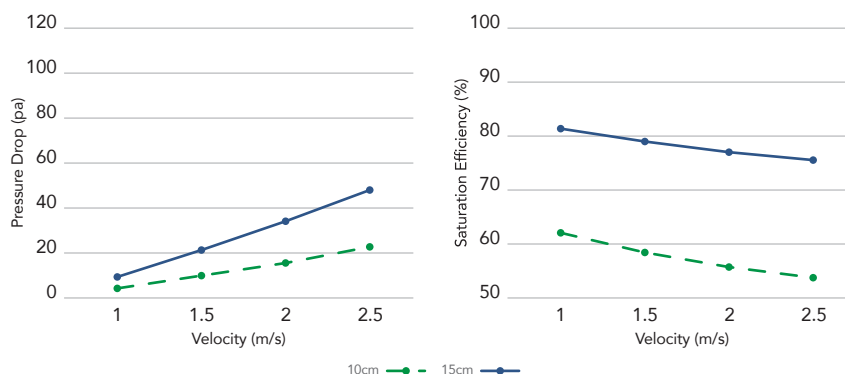
نمودار راندمان و افت فشار سری ۷۰۶۰ (۴۵/۱۵)
