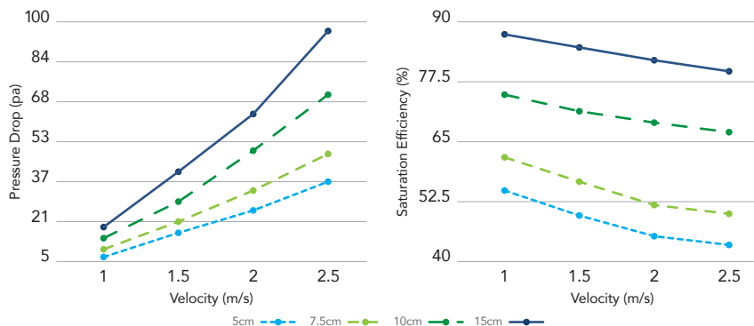
نمودار راندمان و افت فشار سری ۷۰۹۰ (۴۵/۴۵)
