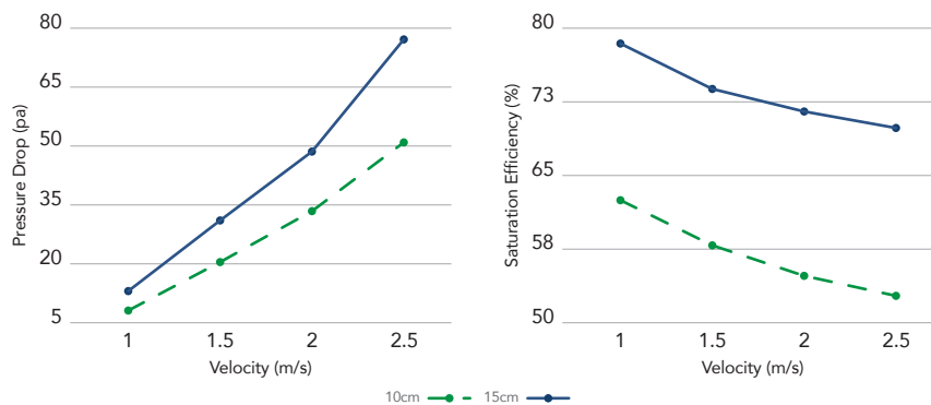
نمودار راندمان و افت فشار سری ۸۰۹۰ (۴۵/۴۵)
