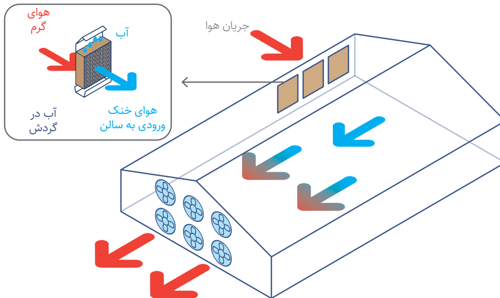
شکل ۱: سیستم پد و فن در مرغداری
